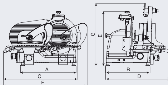
Versione per salumi, version with ham hopper, Ausfuehrung für Wurst, versione pour charcuterie, versión para embutidos
