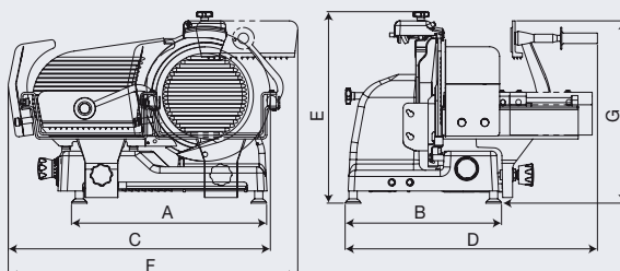
Versione per carni, version with meat hopper, Ausfuehrung für Fleisch, versione pour viandes, versión para carnes
